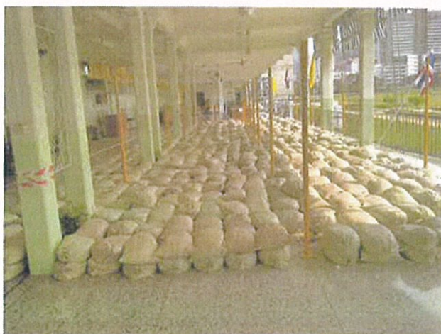
ถุงทรายที่ใช้เป็นน้ำหนักบรรทุกทดสอบ บนพื้นที่ทดสอบ
