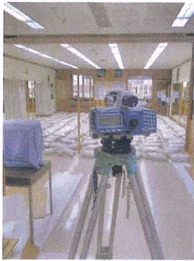
กล้องระดับความละเอียดสูงที่ใช้ตรวจวัดการแอ่นตัวของพื้น
